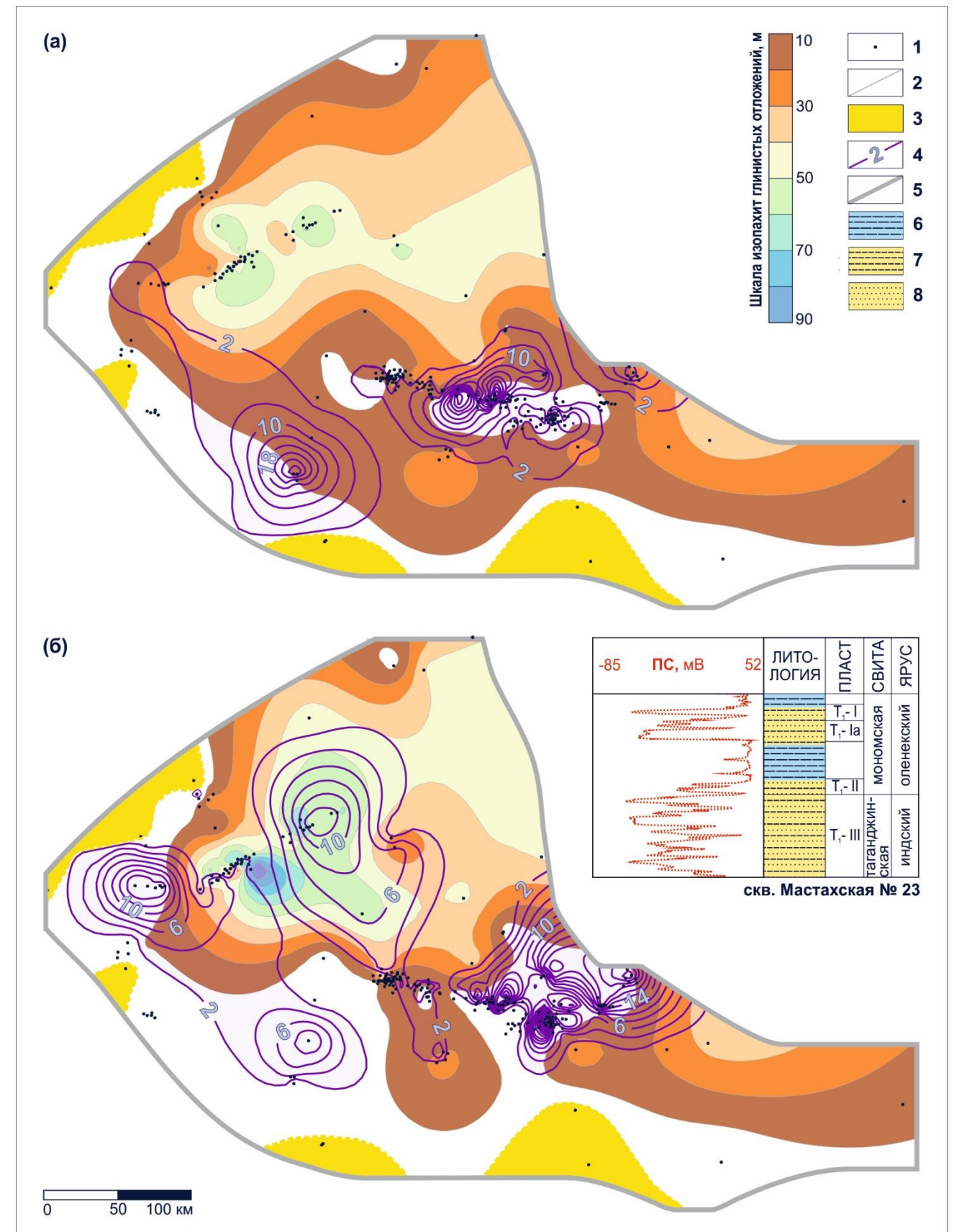
Рисунок 8 – Карты изопакит глинистых пород мономической свиты, перекрывающих песчаные пласты (а) T 1 -I и (б) T 1 -Ia
