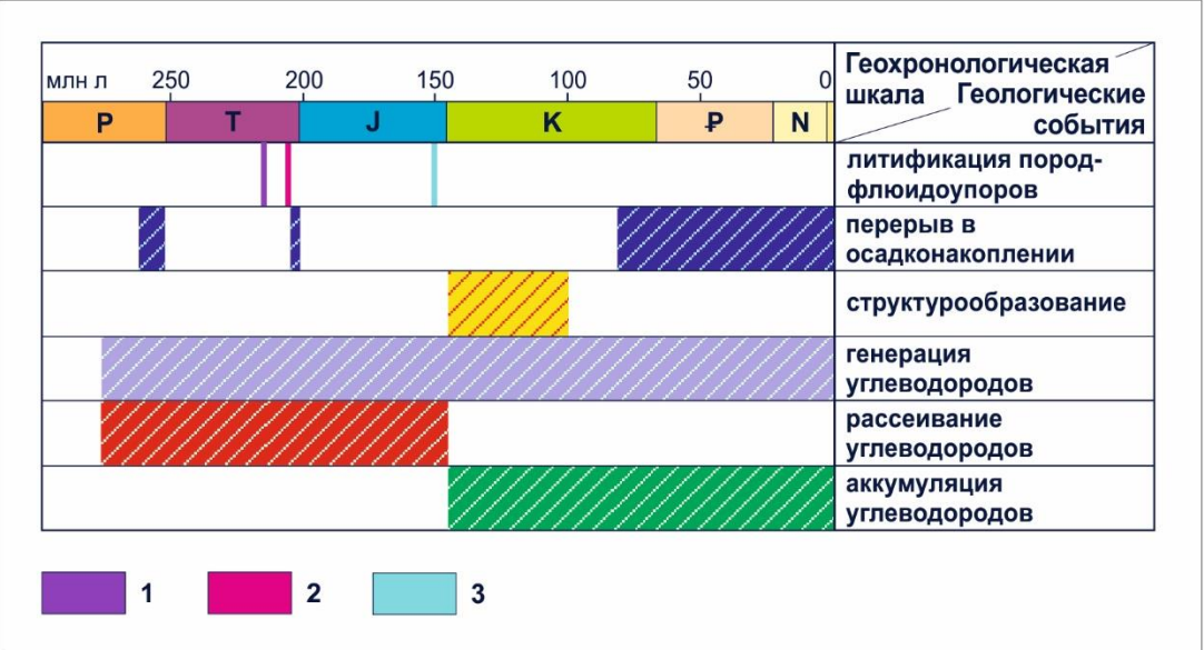
Рисунок 7 – Диаграмма геологических событий для верхнепалеозойско-мезозойской нефтегазовой системы Хапчагайского мегавала Вилуйской гемисинеклизы
