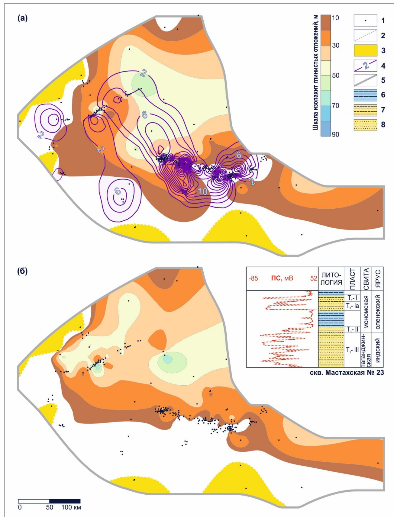
Рисунок 9 – Карты изопакит глинистых пород мономской свиты, перекрывающих песчаные пласты (а) T 1 -II мономской свиты и (б) T 1 -III таганджинской свиты Условные обозначения: см. на рисунке 8.
