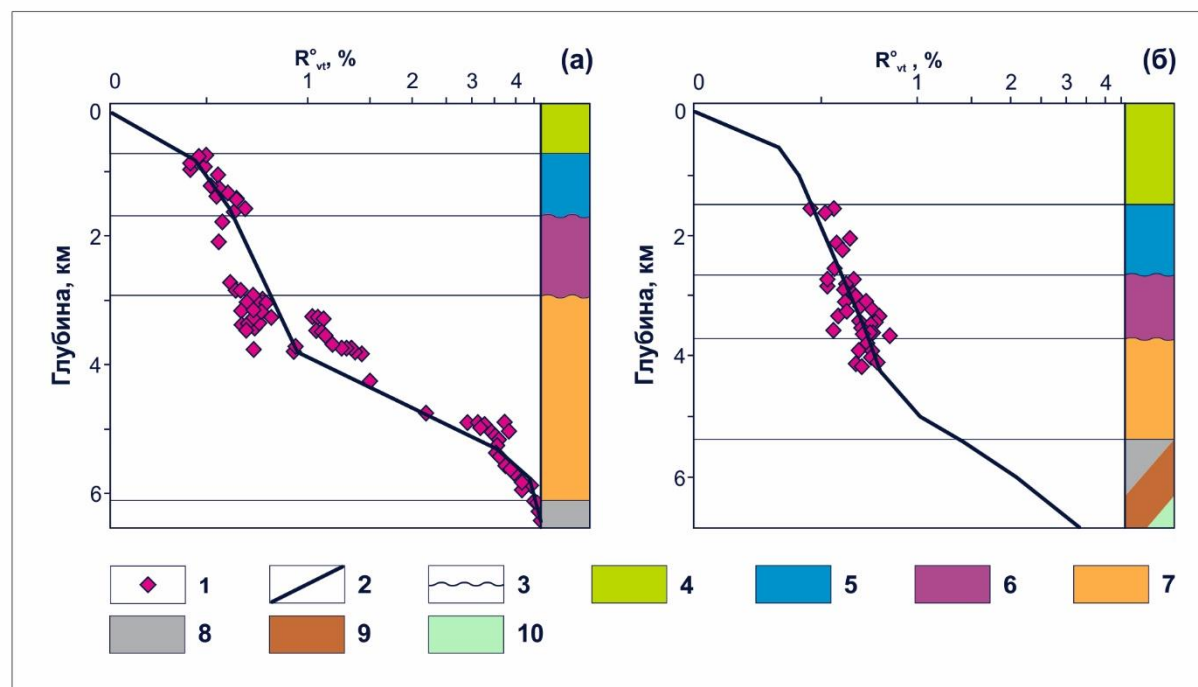
Рисунок 3 – Результаты калибровки плотности теплового потока по отражательной способности витринита на территории (а) Халчагайского мегавала и (б) Логлорского вала
