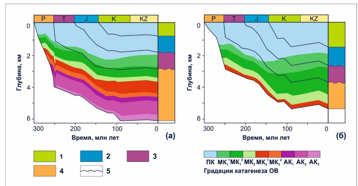
Рисунок 4 – История погружения осадочных комплексов и изменения катагенетической преобразованности ОВ в разрезе скважин (а) Халчагайского мегавала и (б) Логлорского вала в позднепалеозойское, мезозойское и кайнозойское время
