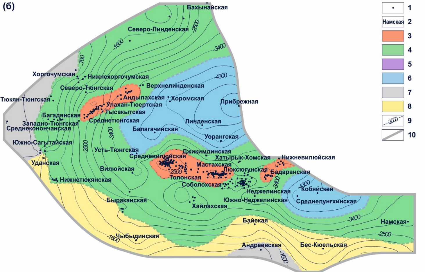
Рисунок 11 – Карты перспектив нефтегазоносности (а) верхнепермского, (б) нижнетриасового и (в) нижнеюрского нефтегазоносных комплексов
