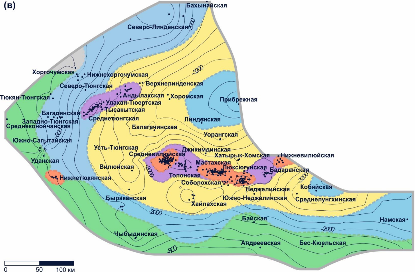
Рисунок 11 – Карты перспектив нефтегазоносности (а) верхнепермского, (б) нижнетриасового и (в) нижнеюрского нефтегазоносных комплексов
